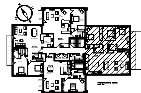
PLAN CLE - 8IEME ETAGE
