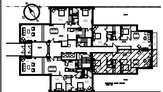
PLAN CLE - REZ-DE-CHAUSSEE
