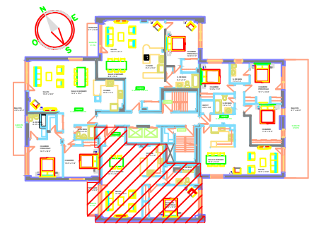
PLAN CLE - 10IEME ETAGE
